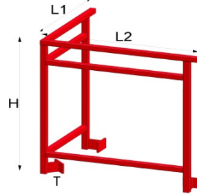
Geländer, Zaunteile ohne Füllung T max. 250mm (L1+L2) \times H L1 max. 600mm
