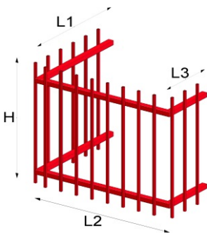
Geländer, Zaunteile mit Füllung (L1+L2+L3) \times H L1 max. 600mm
